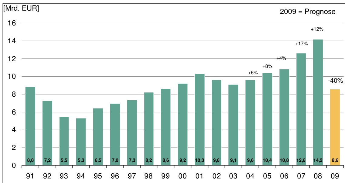
Abb. 2: Werkzeugmaschinenbau in Deutschland: Produktion (in Mrd. Euro)
