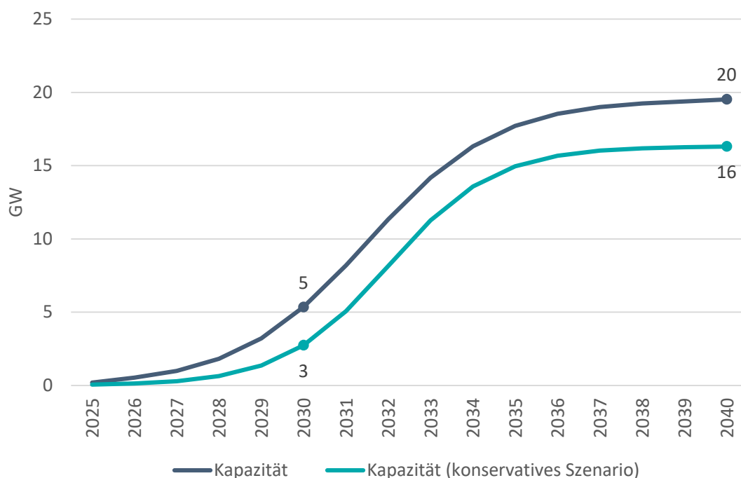
Abbildung 3: Wasserstoffkapazität in Niedersachsen
