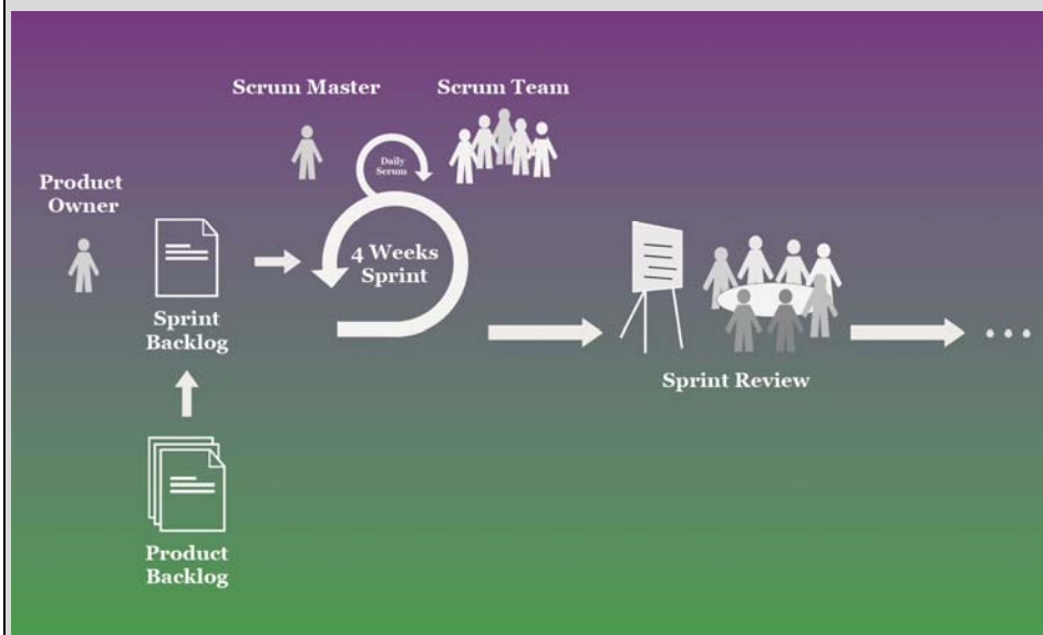
Abb. 1: Der Scrum-Prozess
